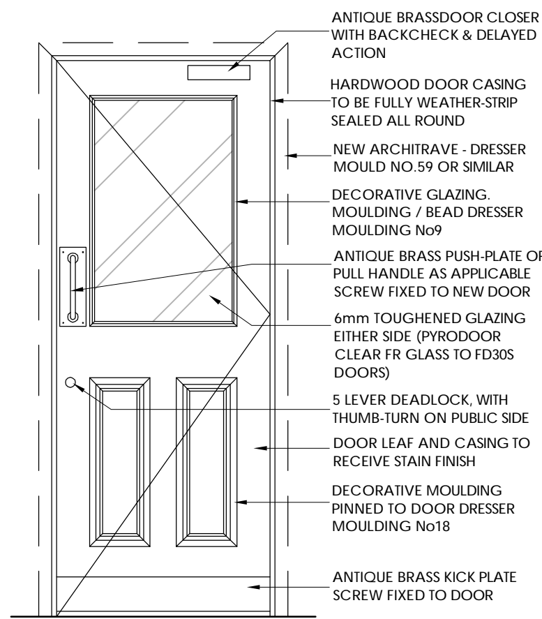
DOOR TYPE F - LOBBY/INTERNAL LINK DOOR
