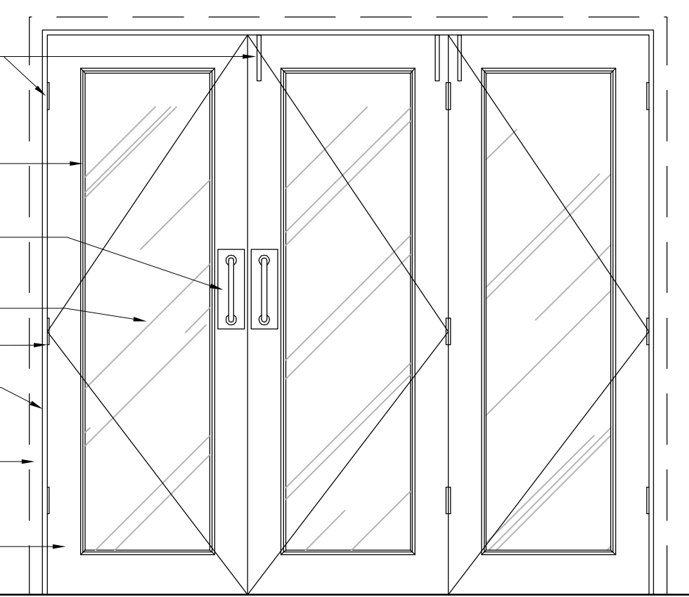
DOOR TYPE G - INTERNAL LINK/SWING DOOR
