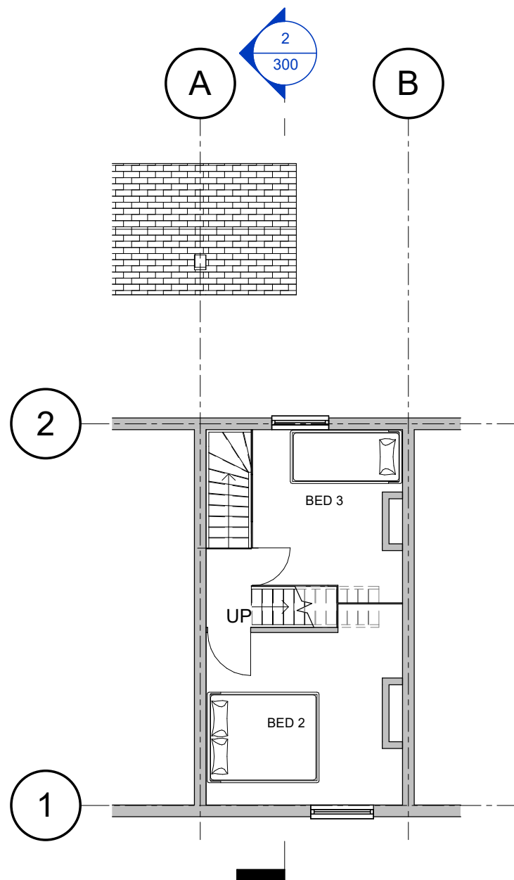
Level 1 - Existing 1 : 100
