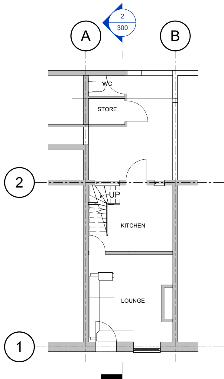
Level 0 - Existing 1 : 100
