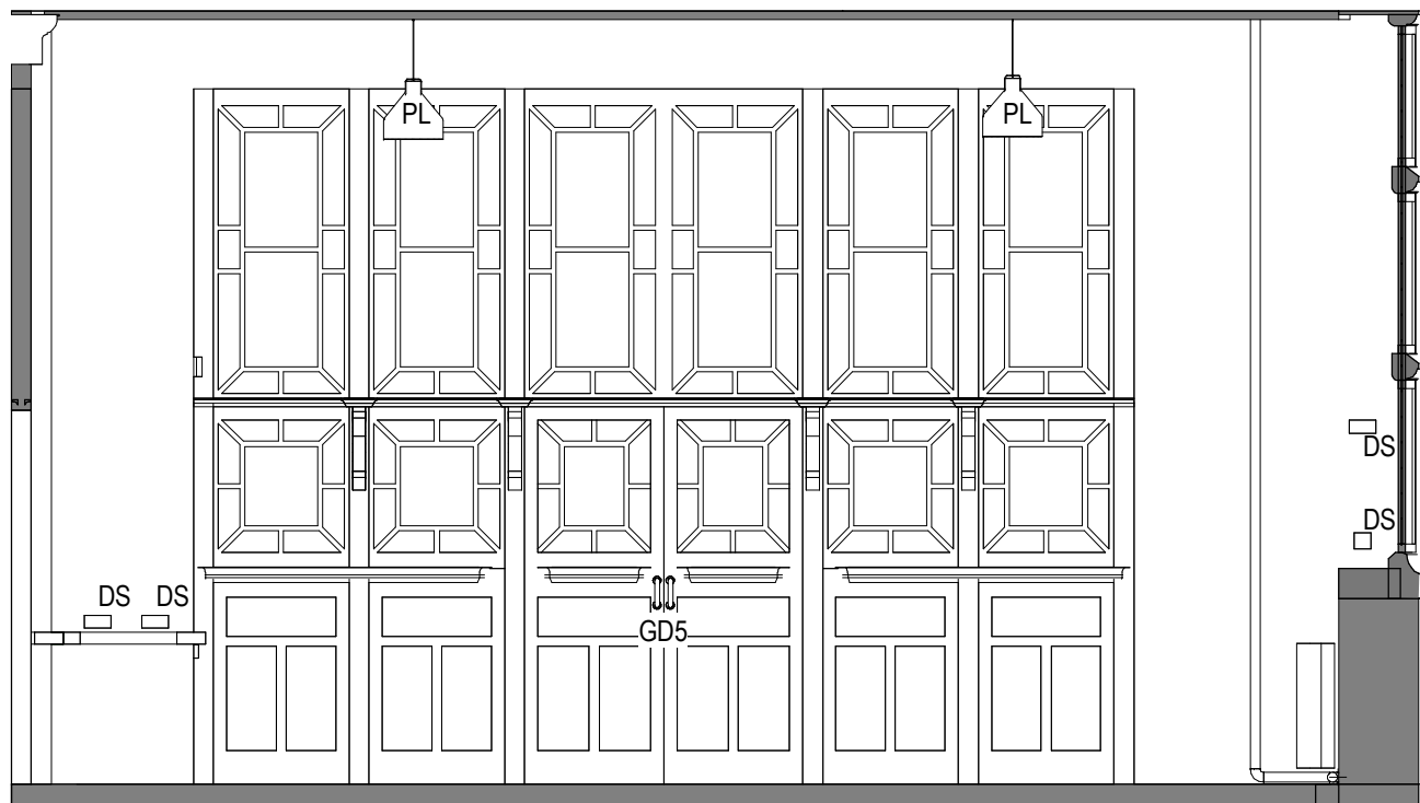
G0005 - Elevation A 1 : 50
