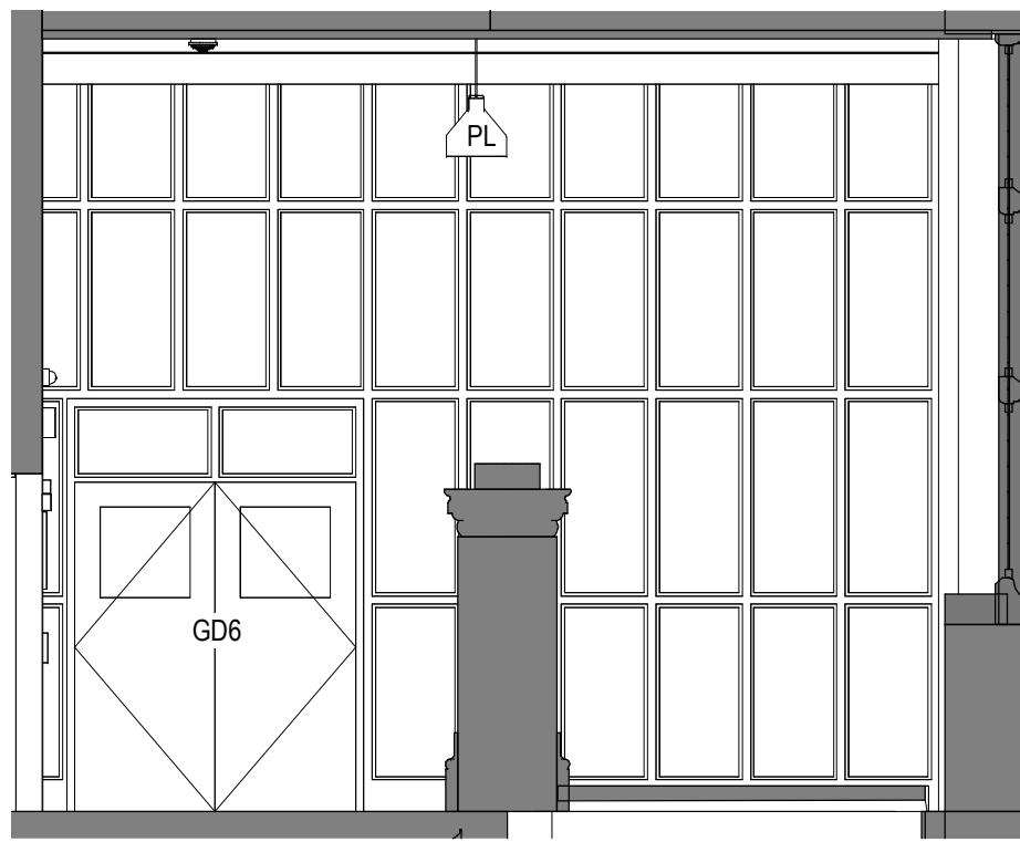
G0009 - Elevation A 1 : 50
