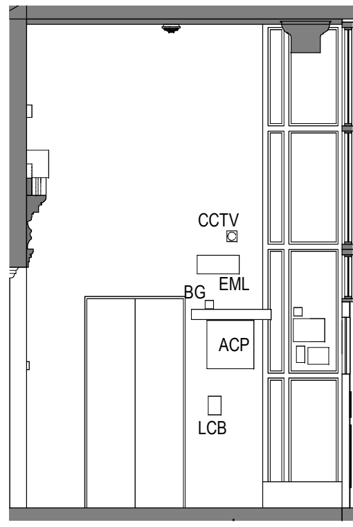
G0009 - Elevation C 1 : 50
