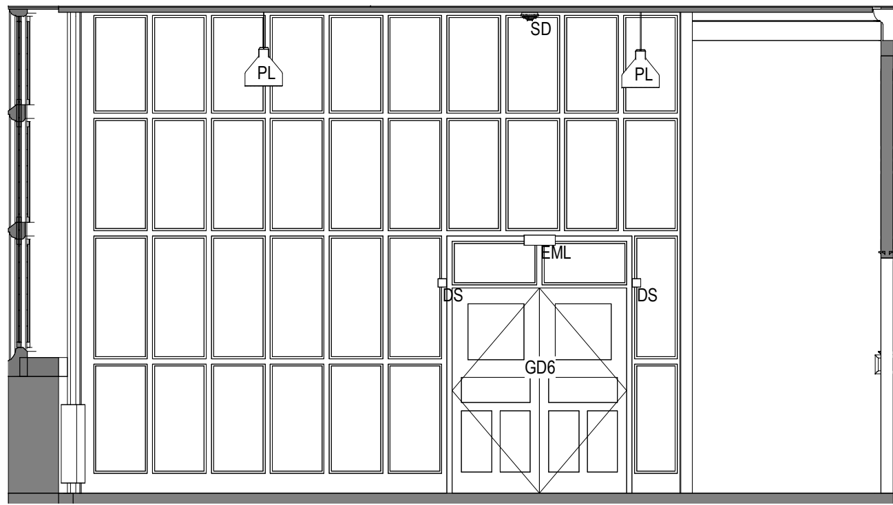
G0005 - Elevation C 1 : 50
