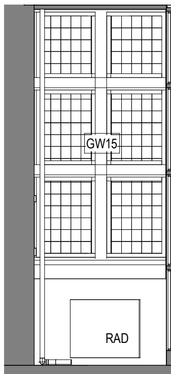
G0005 - Elevation B 1 : 50
