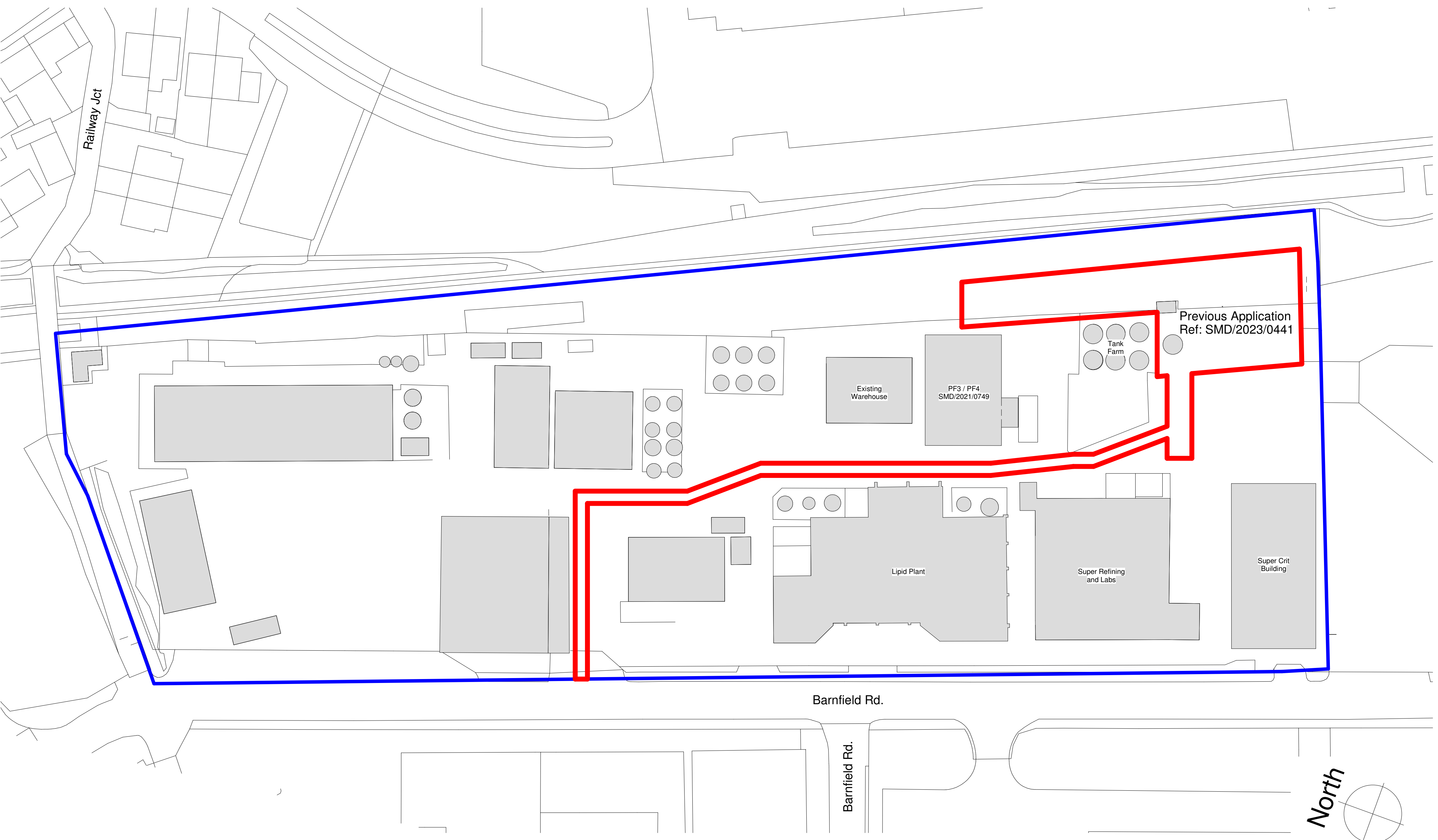
Site Block Plan 1 : 500
