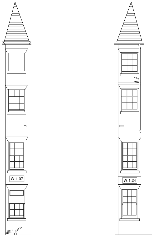
Elevation A
