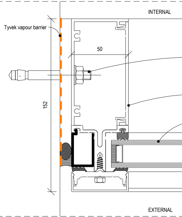
Detail 3: Jamb 1:2
