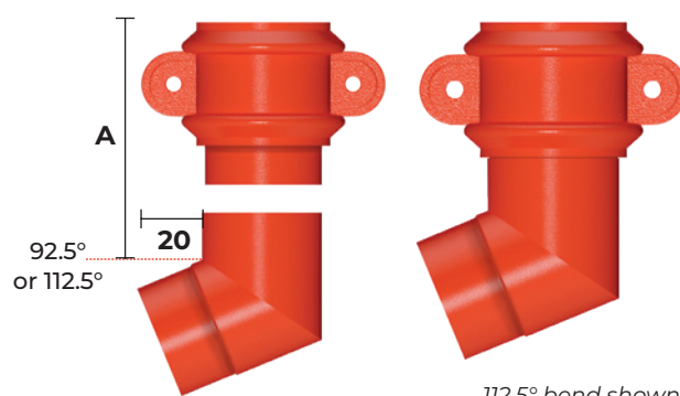
112.5° bend shown
