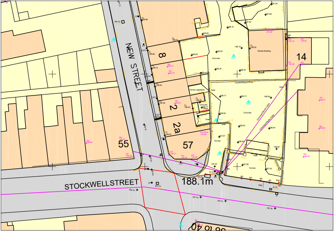
Site Plan - 1:500
