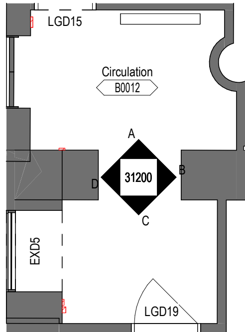
Callout Plan 1 : 50
