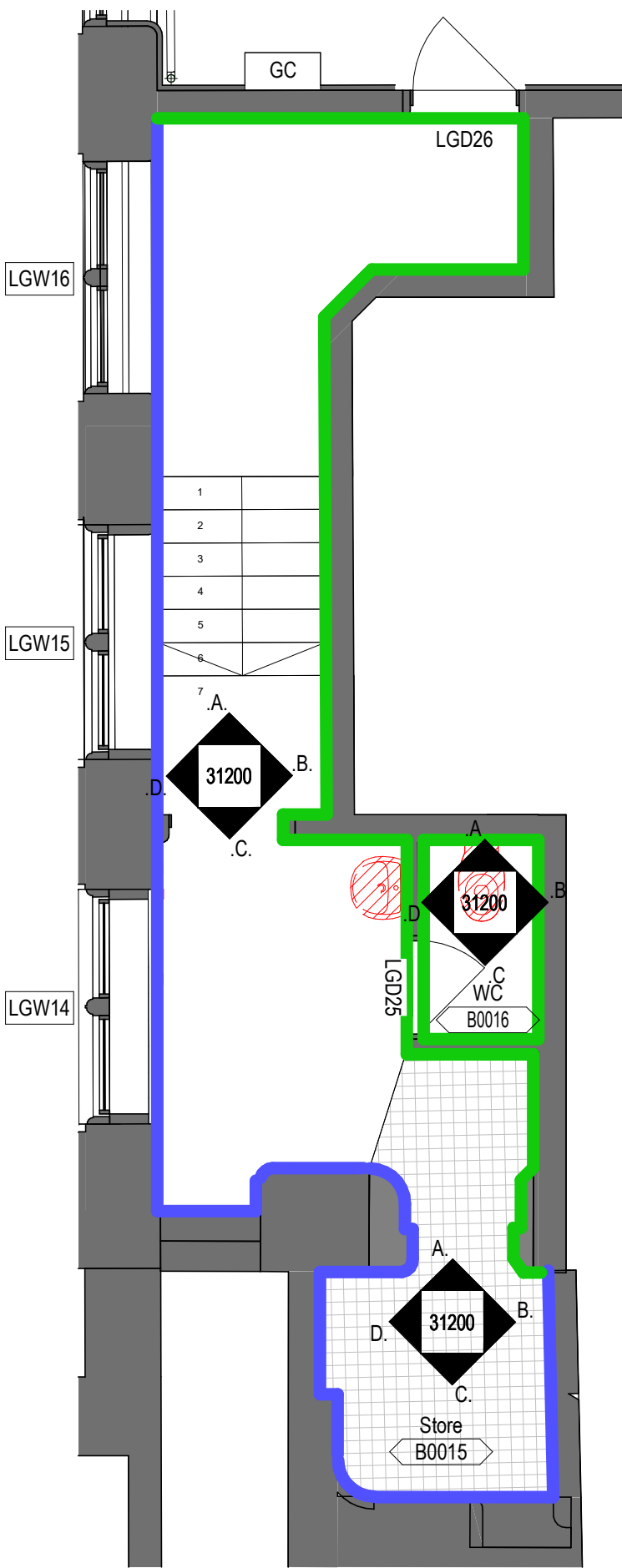
Callout Plan 1 : 50
