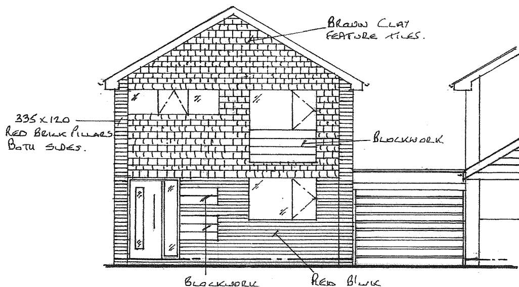
EXT'G FRONT ELEVATION
