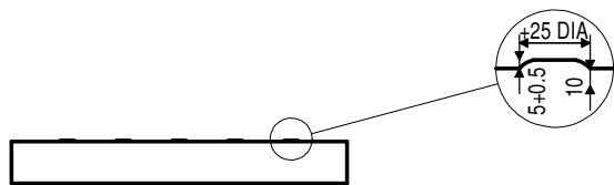
Elevation
