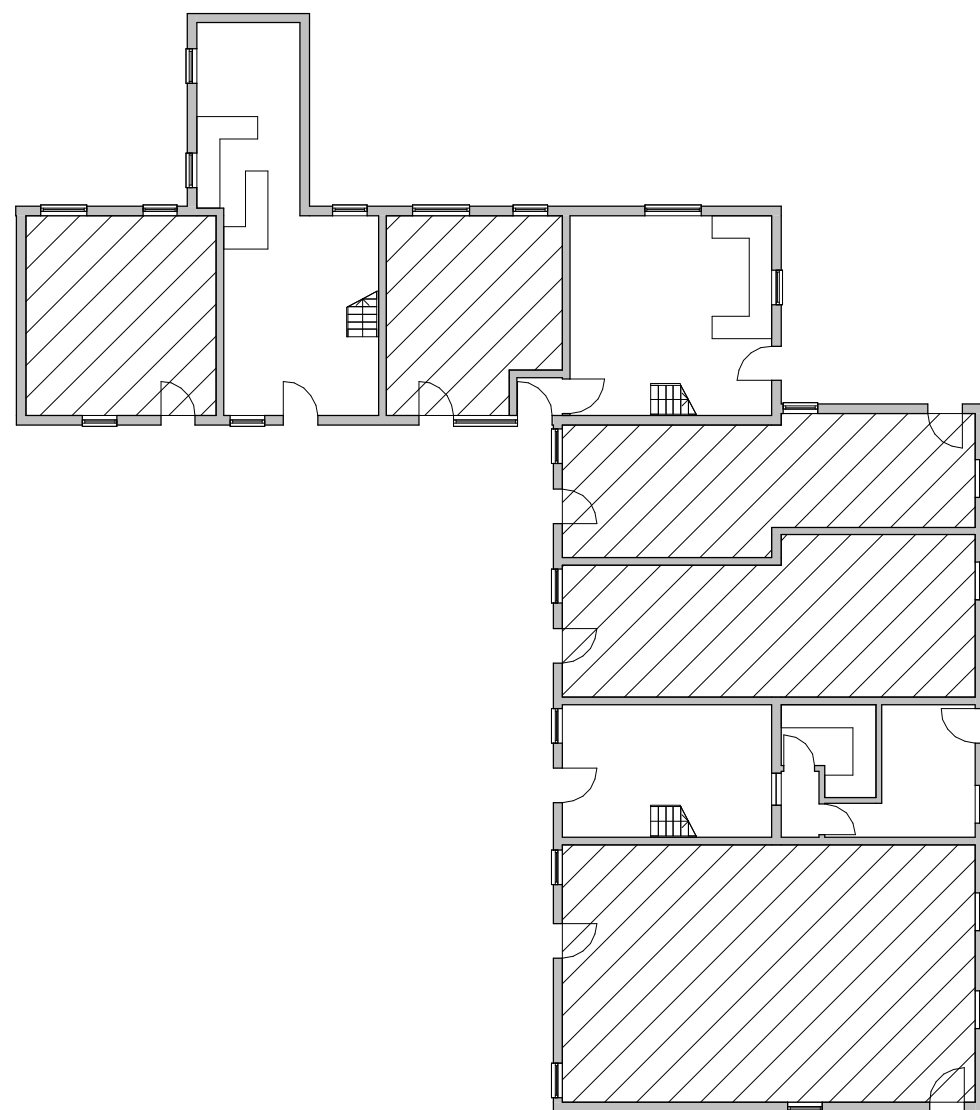
1 Level 0 1 : 200
