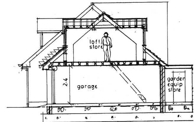
1:50 SECTION A-A
