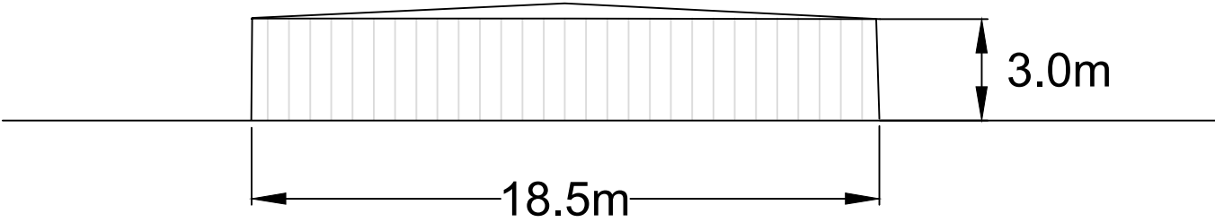
ELEVATION
