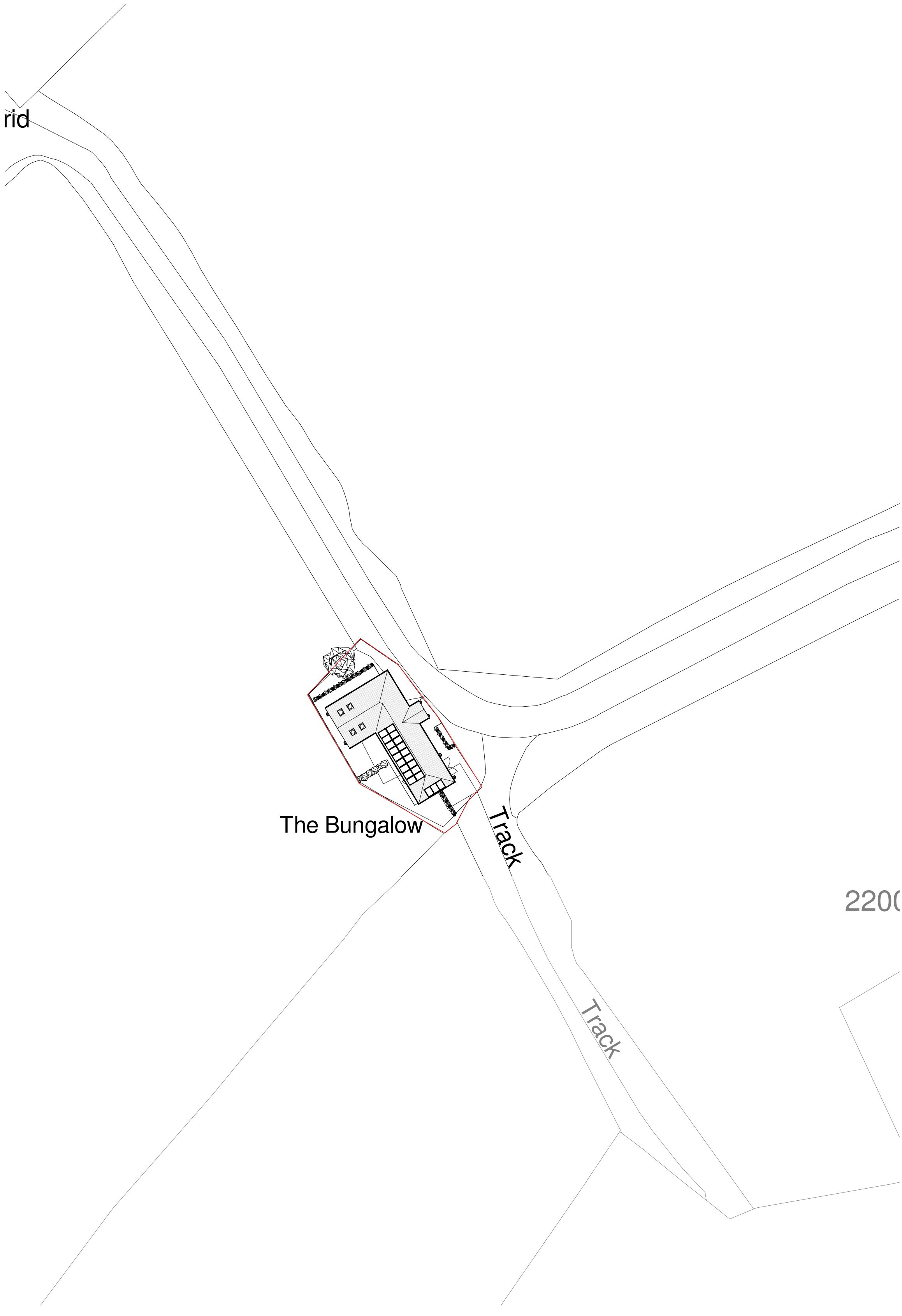
Block Plan 1 : 500
