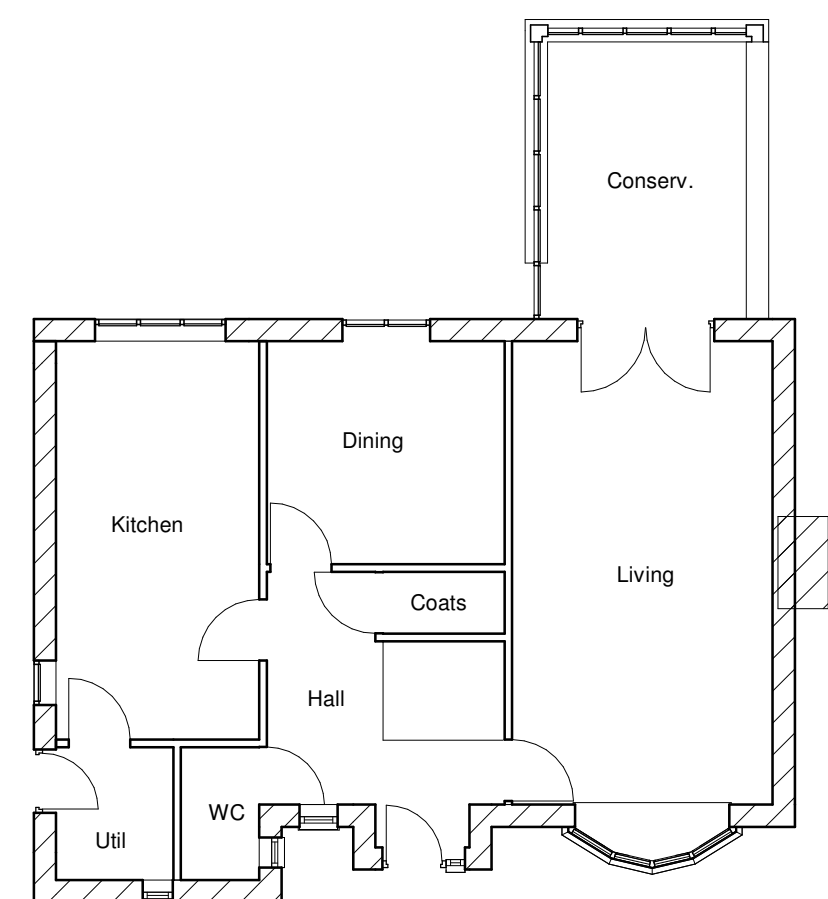
GFL Existing 1 : 100
