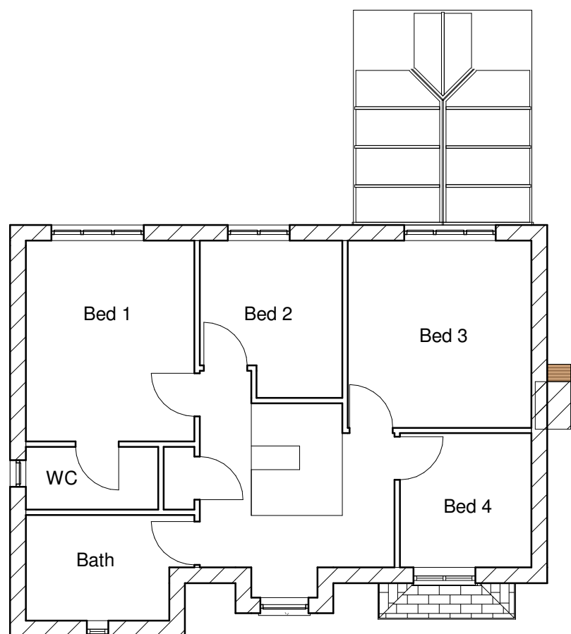
FFL Existing 1 : 100
