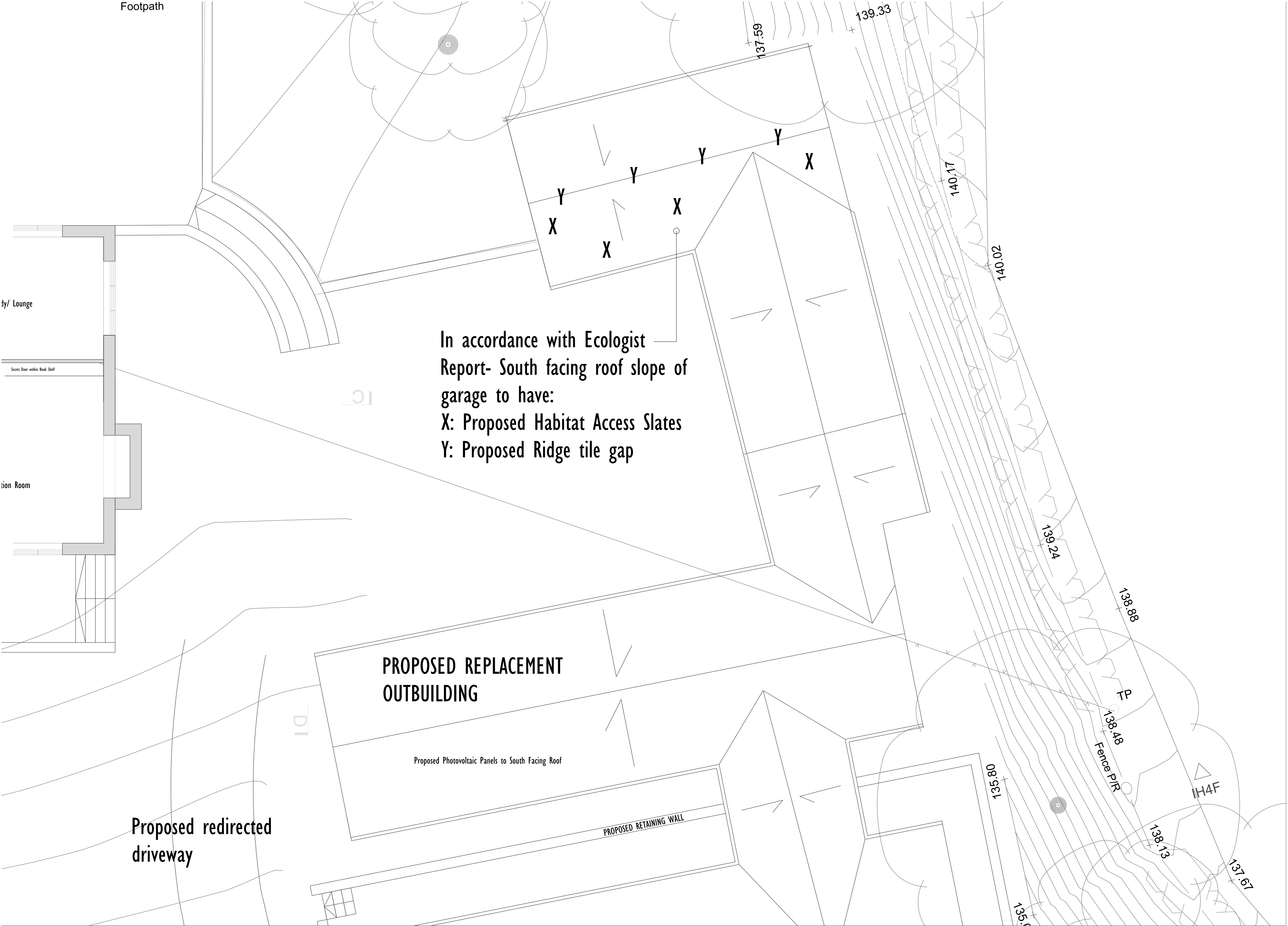
Site Plan (1:50)
