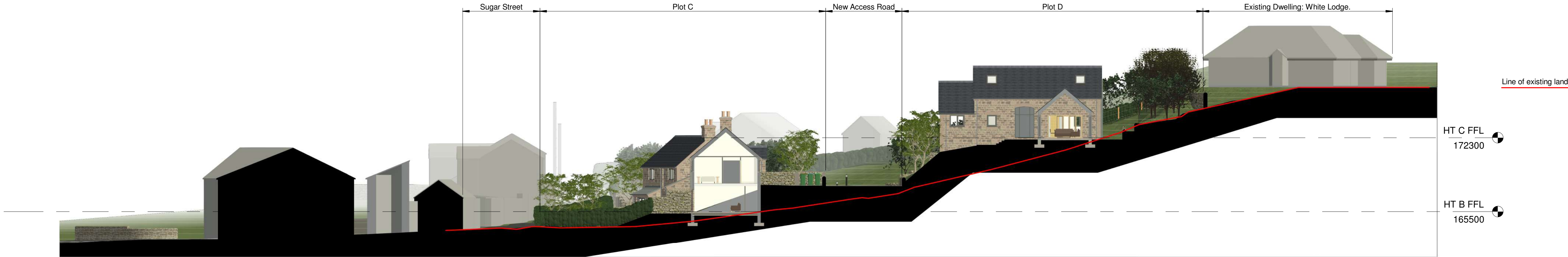
Section 1 1 : 200
