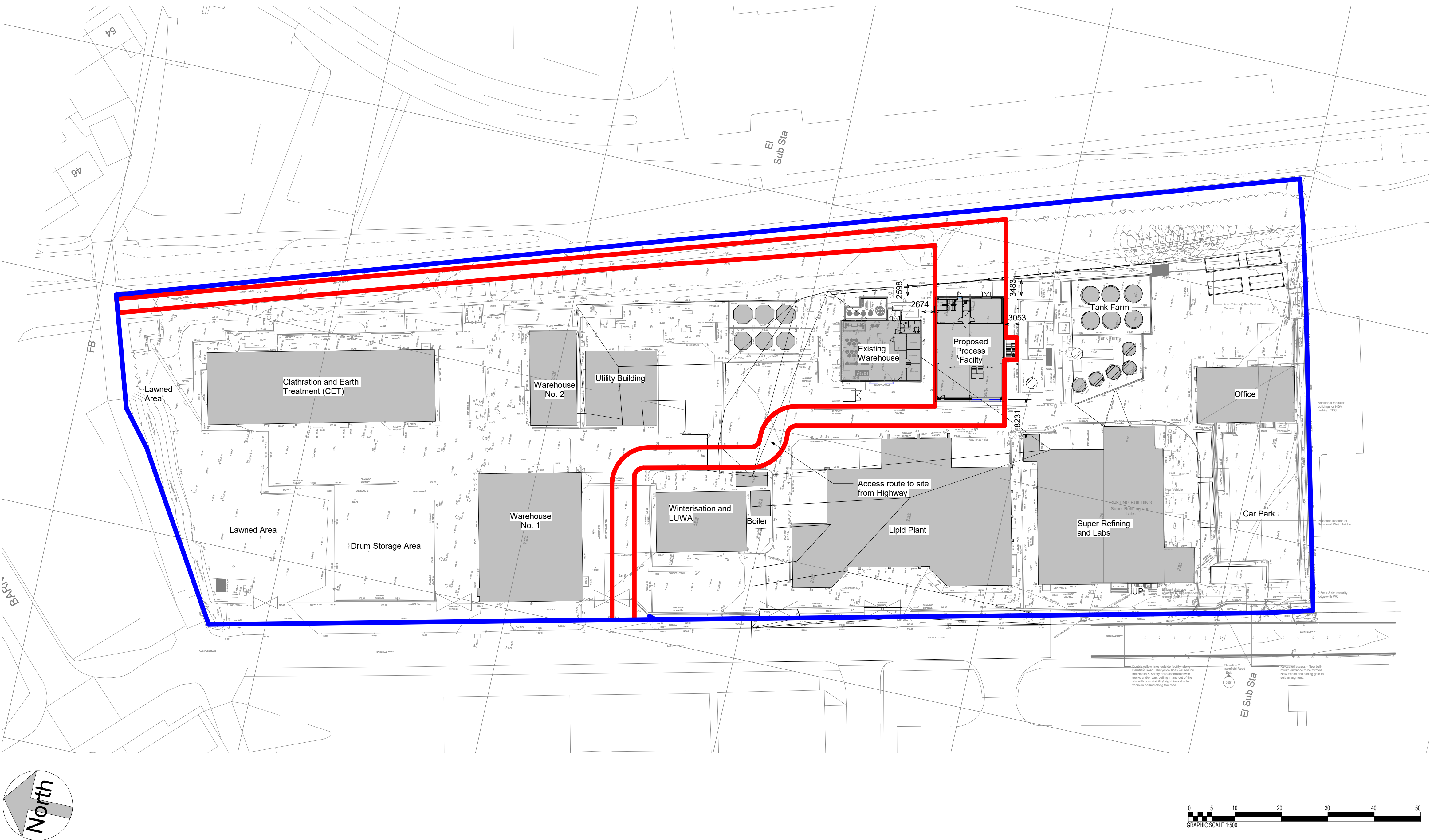
1 Site Block Plan 1 : 500
