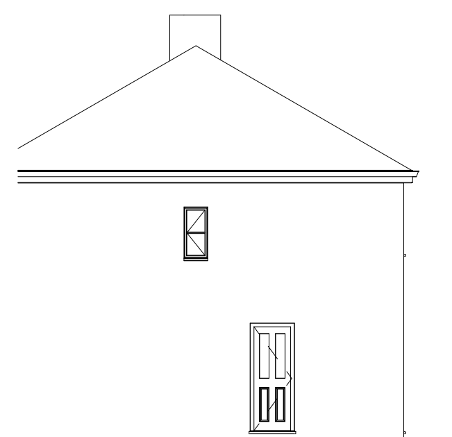
8 Side Existing 1 : 100
