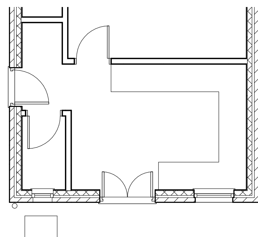
1 GFL Existing 1 : 50
