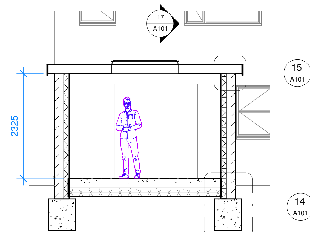
13 Section 1 1 : 50
