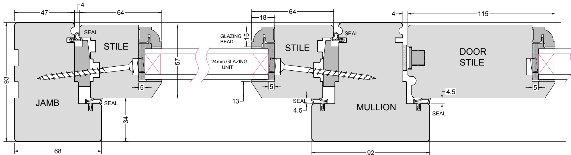
SECTION A-A
