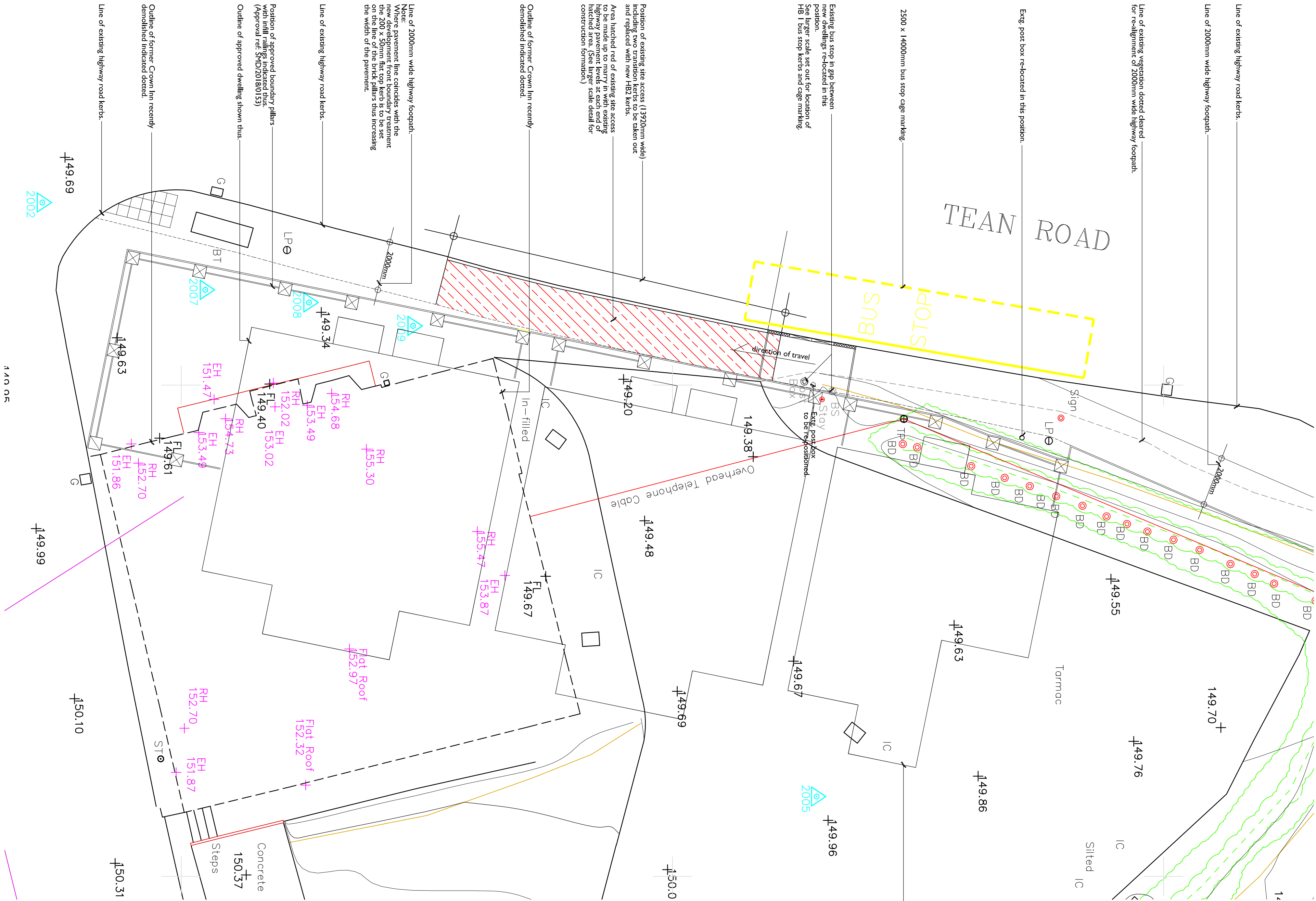
Plan layout scale: 1:100 at A1
