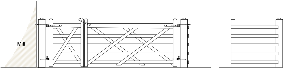
Elevation A
