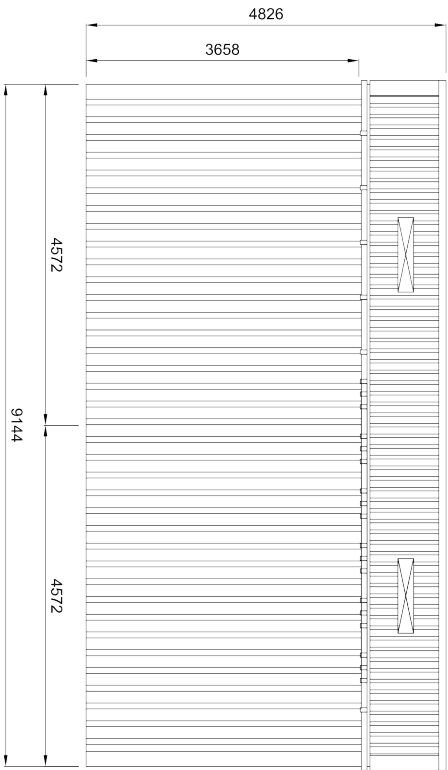
ELEVATION B
