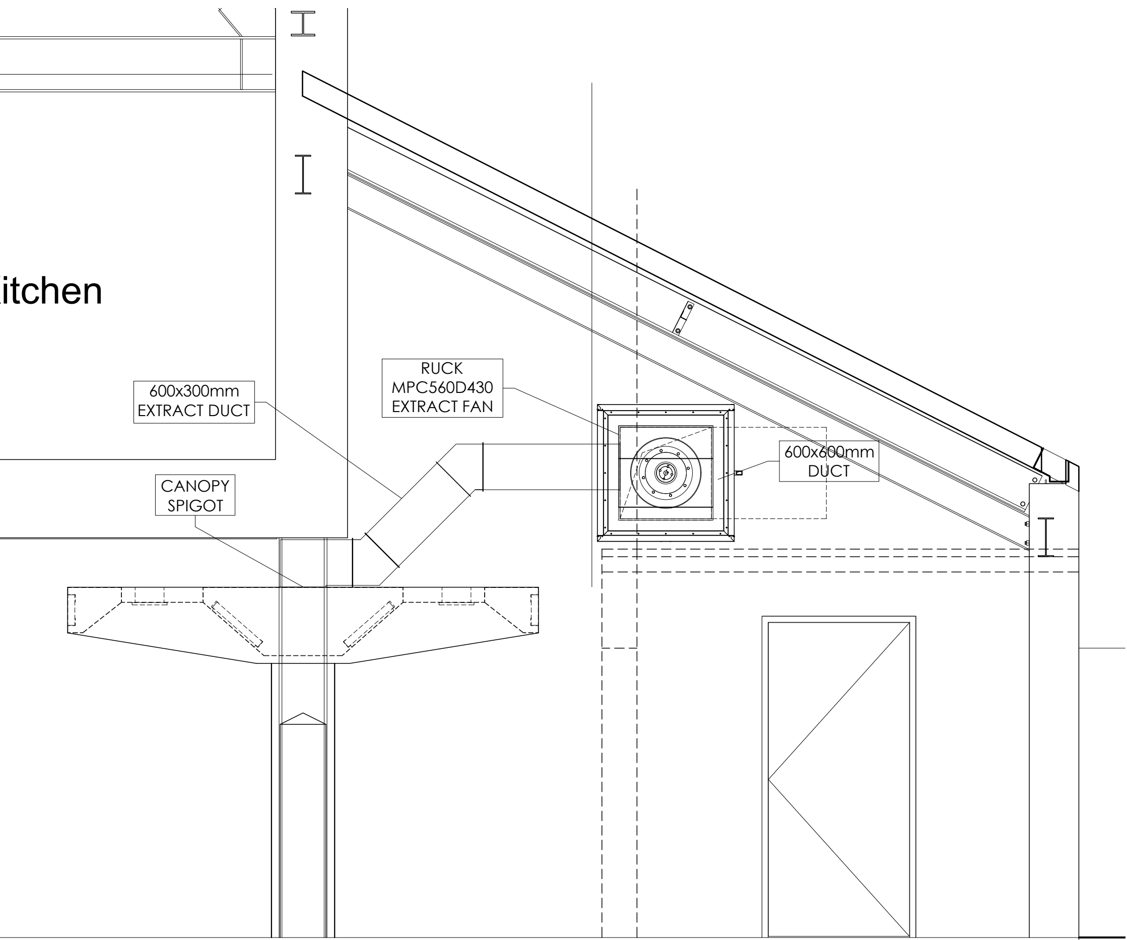
ELEVATION B-B
