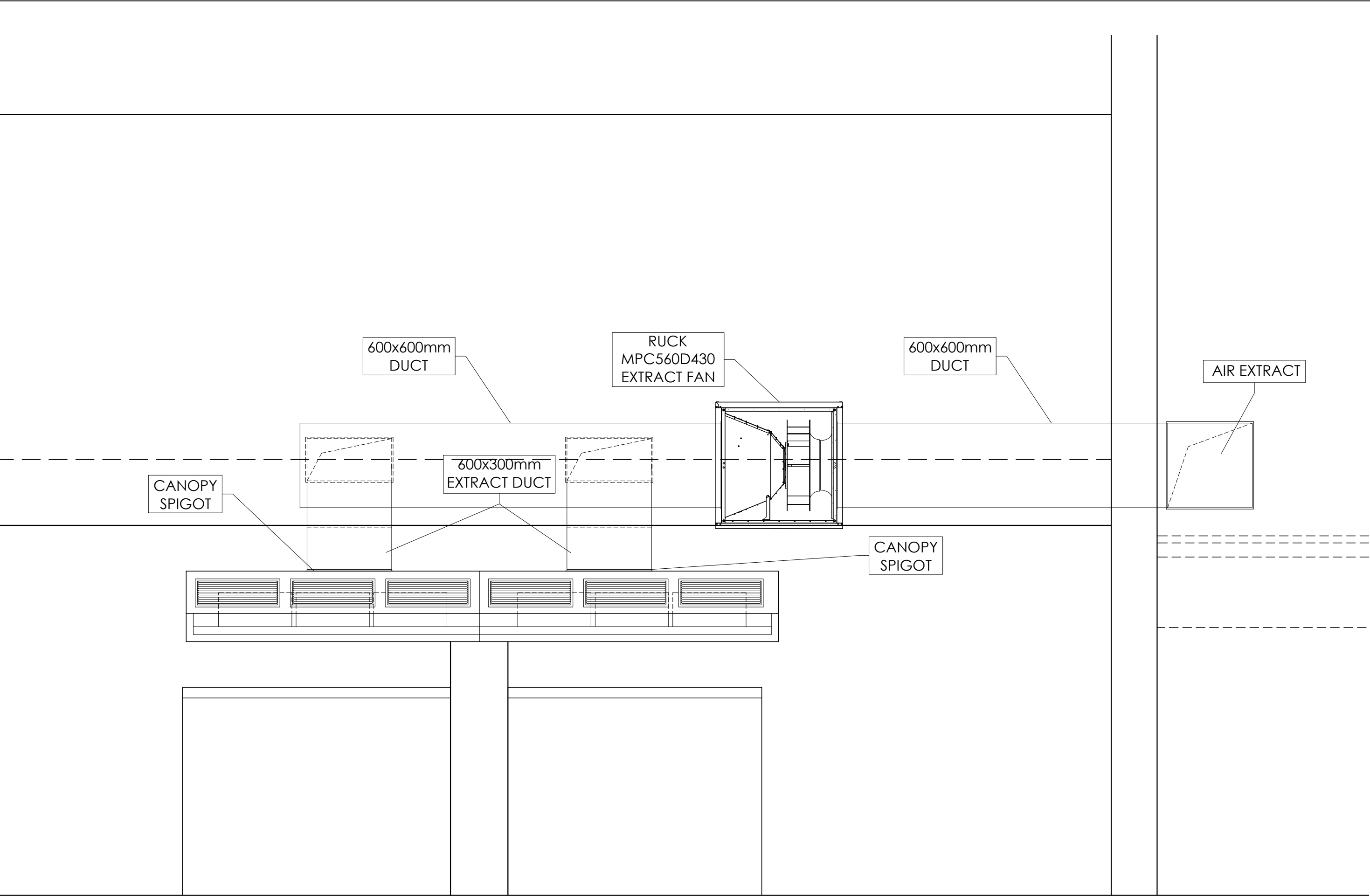
ELEVATION A-A
