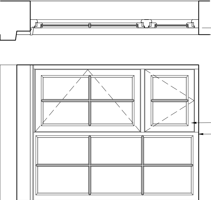
VERT SECTION
