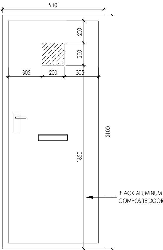
DOOR ELEVATION Scale 1:20
