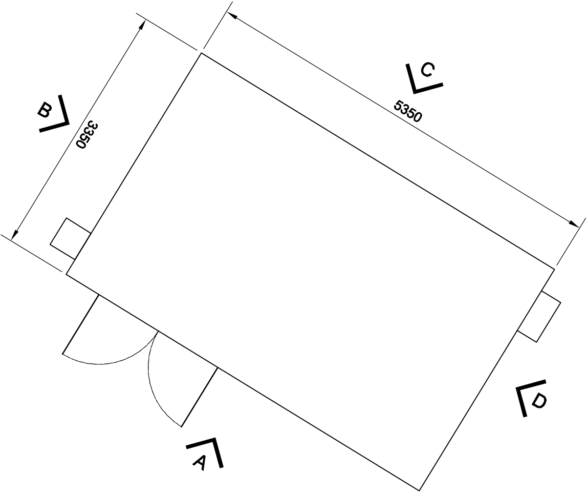
Plan of PO4 Kiosk 1:50
