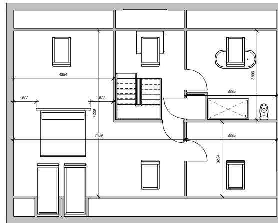
3 House Floor 2 1 : 50
