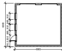
8 Garage FFL 1 : 100
